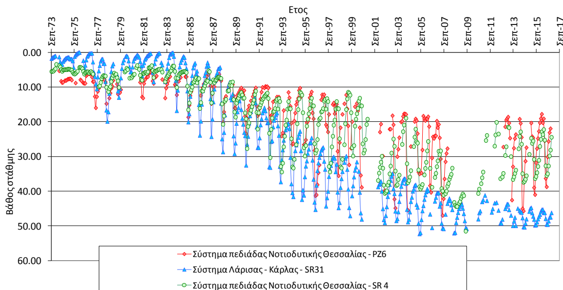
Διακύμανση στάθμης πιεζομέτρων - Συσχέτιση με περίοδο ξηρασίας 1988-90
