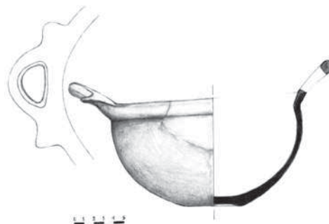
Εικ. 5. Καλαθόσχημος σκύφος με αποφύσεις στις λαβές (Σχέδιο: Ε. Ρίνη).
