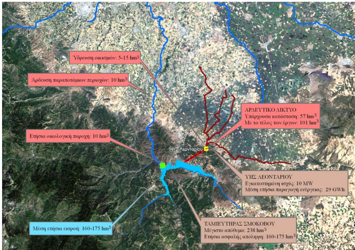
Σχήμα 3.2: Υδροσύστημα Σμοκόβου.
