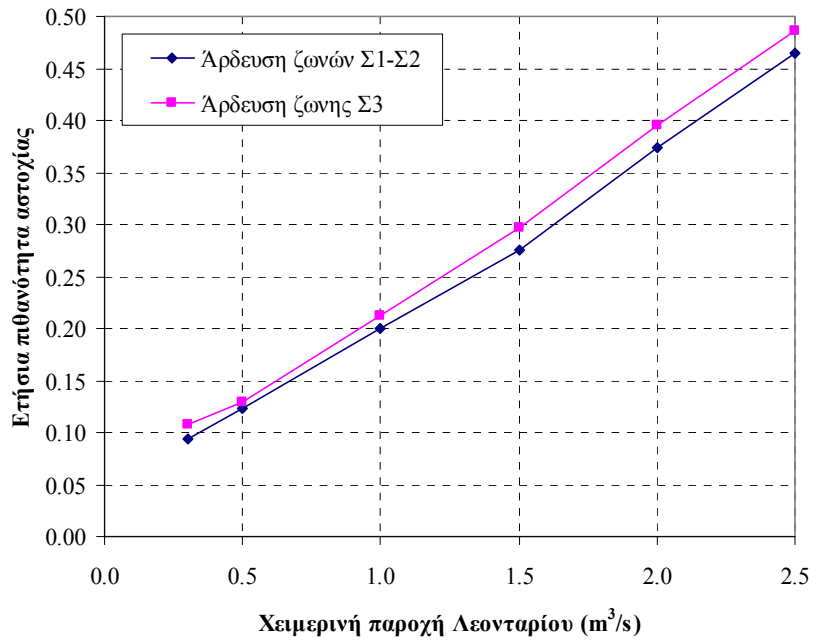
Σχήμα 6.7: Πιθανότητα αστοχίας αρδευτικών στόχων, συναρτήσεως της χειμερινής παροχής του ΥΗΣ Λεονταρίου, με βάση τα σενάρια υψηλής αρδευτικής κατανάλωσης (Γ1).
