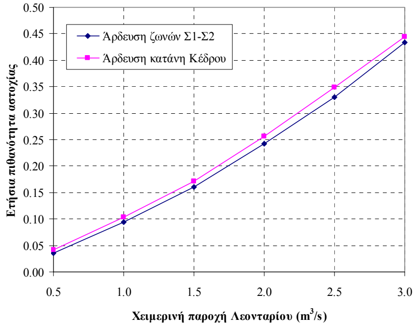
Σχήμα 6.5: Πιθανότητα αστοχίας αρδευτικών στόχων, συναρτήσσει της χειμερινής παροχής του ΥΗΣ Λεονταρίου, με βάση τα σενάρια υψηλής αρδευτικής κατανάλωσης (B1).
