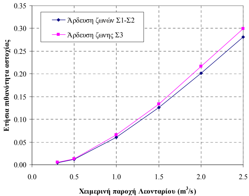
Σχήμα 6.8: Πιθανότητα αστοχίας αρδευτικών στόχων, συναρτήσεως της χειμερινής παροχής του ΥΗΣ Λεονταρίου, με βάση τα σενάρια χαμηλής αρδευτικής κατανάλωσης (Γ2).
