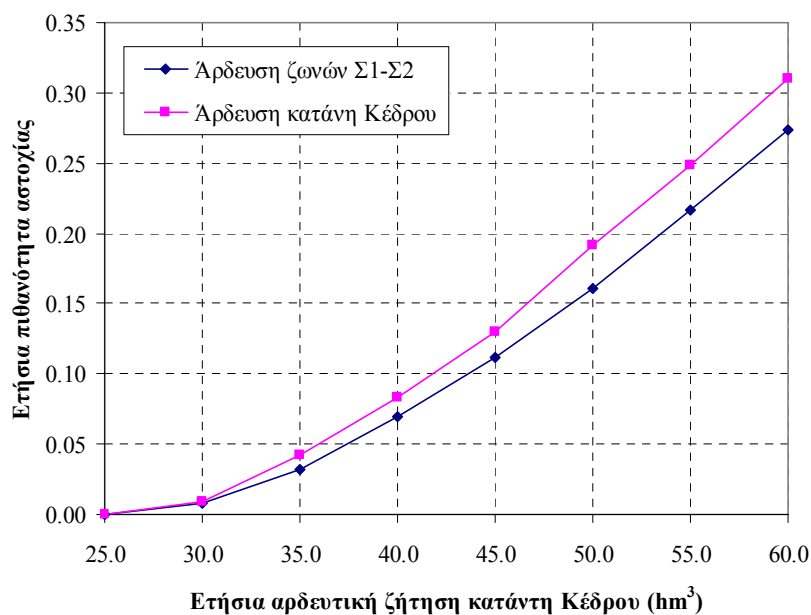
Σχήμα 6.4: Πιθανότητα αστοχίας αρδευτικών στόχων, συναρτήσει της ετήσιας αρδευτικής ζήτησης κατάντη του Κέδρου, με βάση τα σενάρια χαμηλής αρδευτικής κατανάλωσης (A2).
