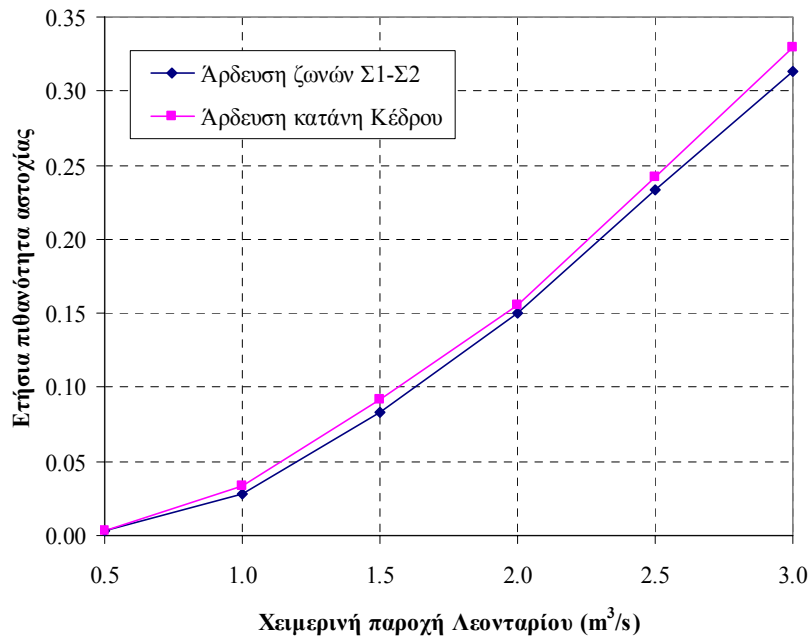
Σχήμα 6.6: Πιθανότητα αστοχίας αρδευτικών στόχων, συναρτήσσει της χειμερινής παροχής του ΥΗΣ Λεονταρίου, με βάση τα σενάρια χαμηλής αρδευτικής κατανάλωσης (B2).
