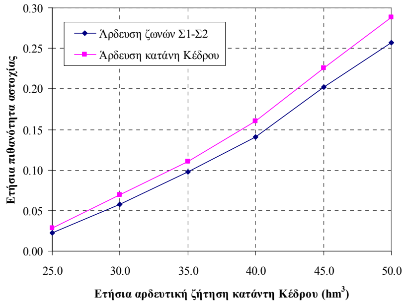
Σχήμα 6.3: Πιθανότητα αστοχίας αρδευτικών στόχων, συναρτήσει της ετήσιας αρδευτικής ζήτησης κατάντη του Κέδρου, με βάση τα σενάρια υψηλής αρδευτικής κατανάλωσης (A1).
