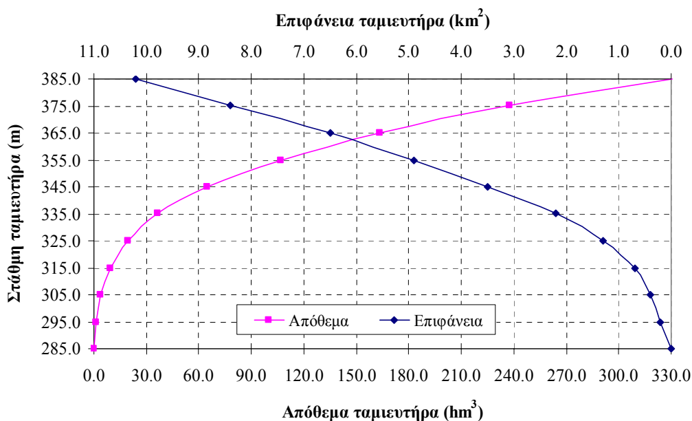
Σχήμα 4.4: Καμπύλες στάθμης-αποθέματος και στάθμης-επιφάνειας ταμιευτήρα Σμοκόβου.
