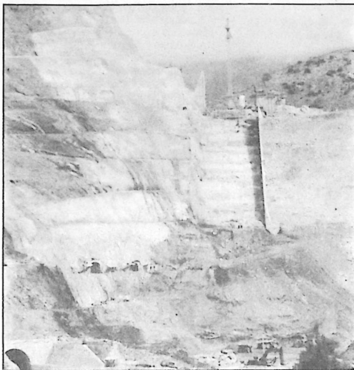
Μερική όψη του φράγματος της Μεσοχώρας — έργο κεφαλής της εκτροπής του Αχελώου
