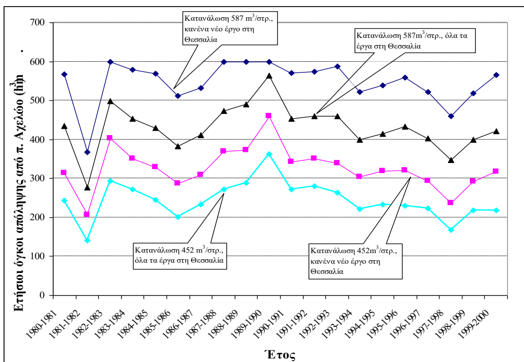
Σχήμα 6.Ετήσιες απολήψεις από τον Αχελώο για διαφορετικά σενάρια. Προέκυψαν από την εφαρμογή του μοντέλου με την υπόθεση ότι θα επαναλαμβάνονταν οι υδρολογικές συνθήκες τις εικοσαετίας 1980-2000.
